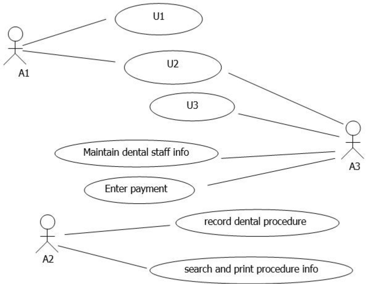
图 3-1 用例图
