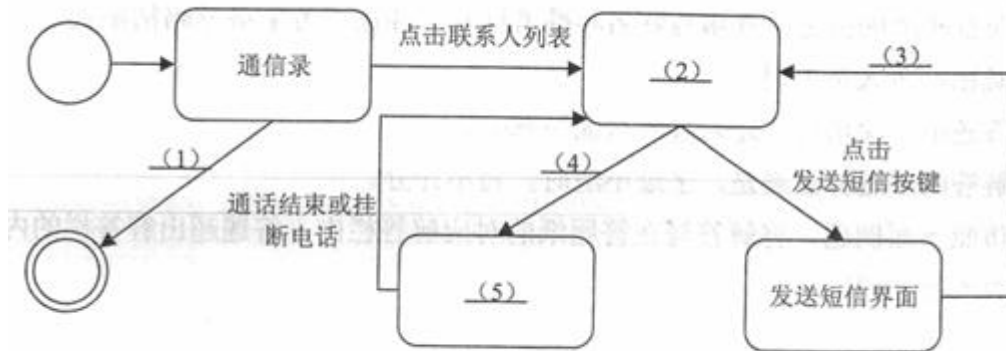
图 2-2 手机通信录管理软件状态机模型
