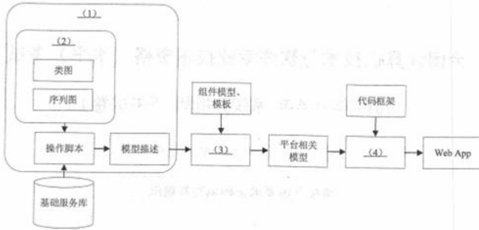
图 2-1 基于 MDA 的软件开发流程
