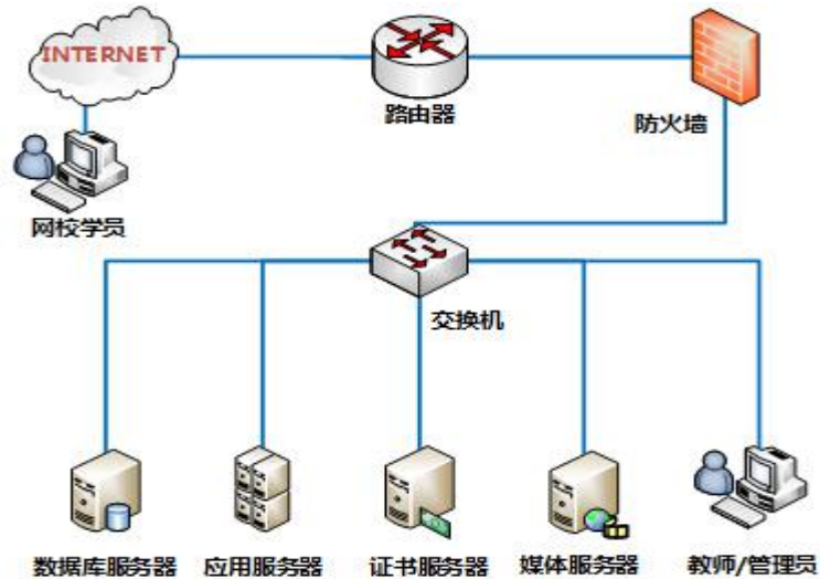
图 4-1 在线网络学校系统拓扑结构
